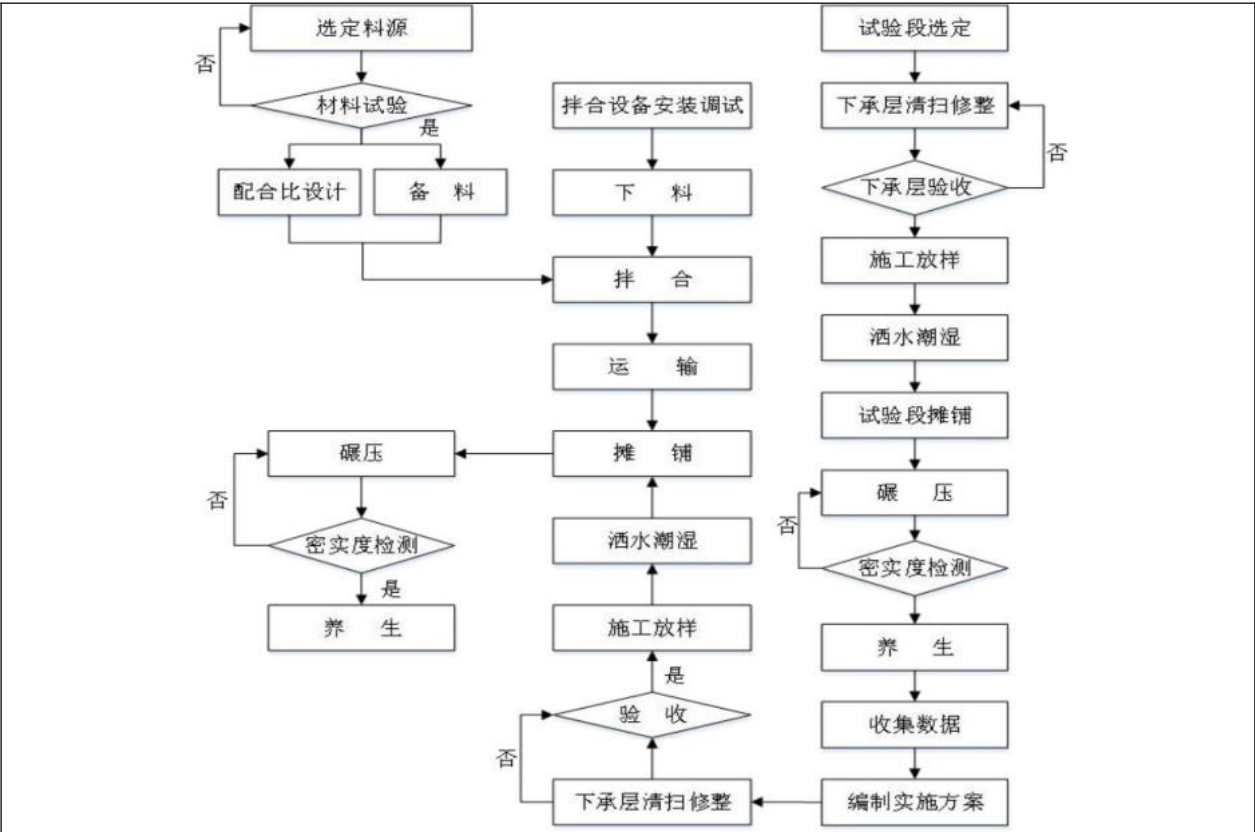
图 4-2 级配碎石路基填筑施工工艺流程图
