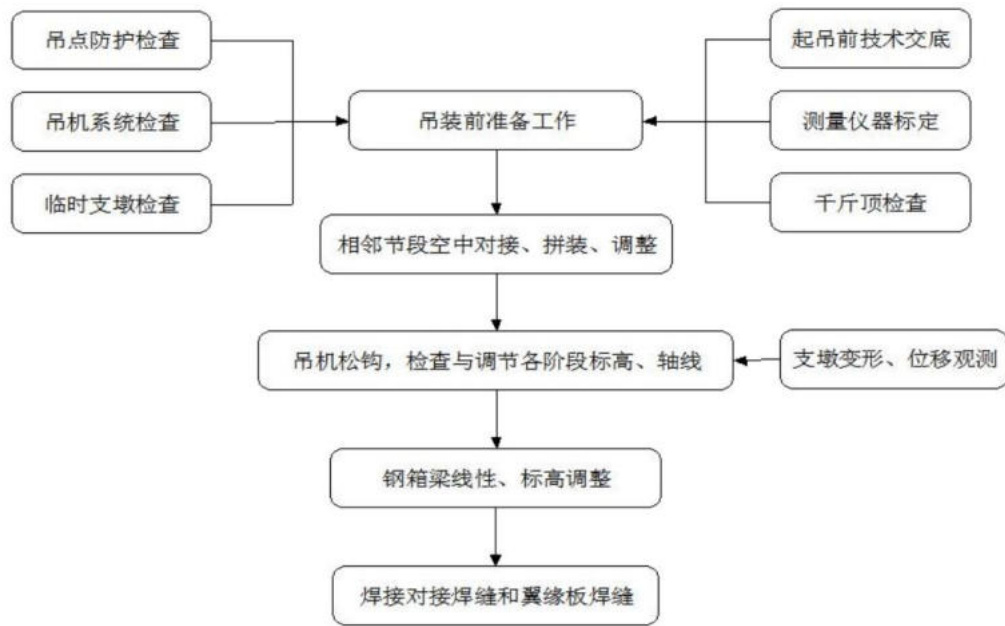
图 4-4 钢箱梁吊装工艺流程图
