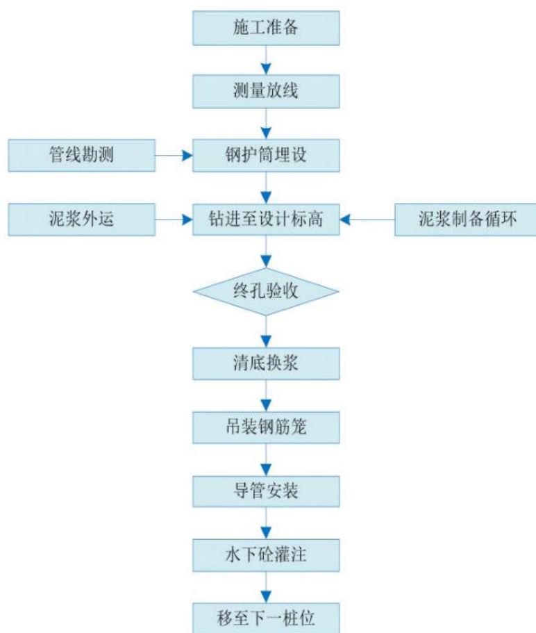
图 4-3 钻孔灌注桩施工工艺流程图
