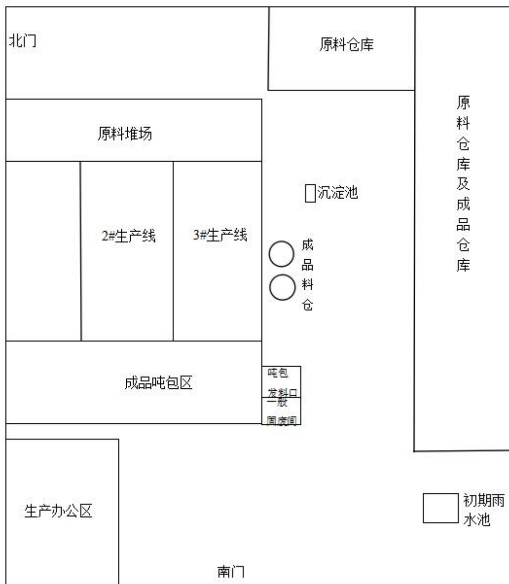
图 2.1-2 项目平面布置图
